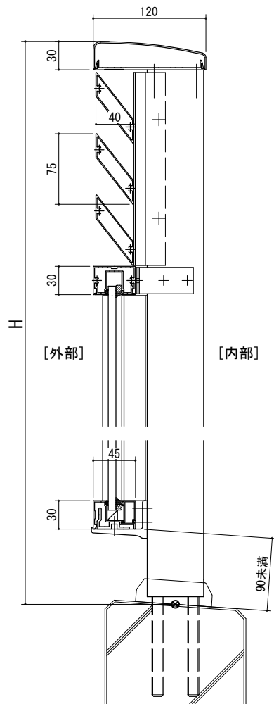
[上ルーバー下ガラス (堅枠A) タイプ]
