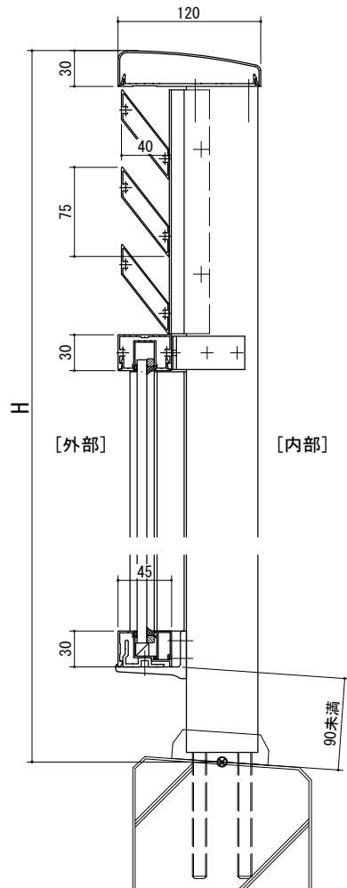
〔上ルーバー下ガラス（竖枠B）タイプ〕
