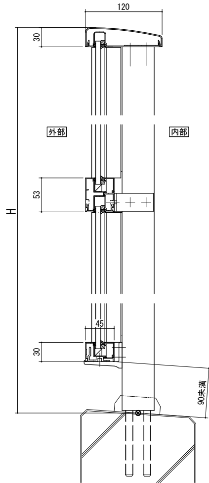
[上下ガラス堅枠Aタイプ] 中間
