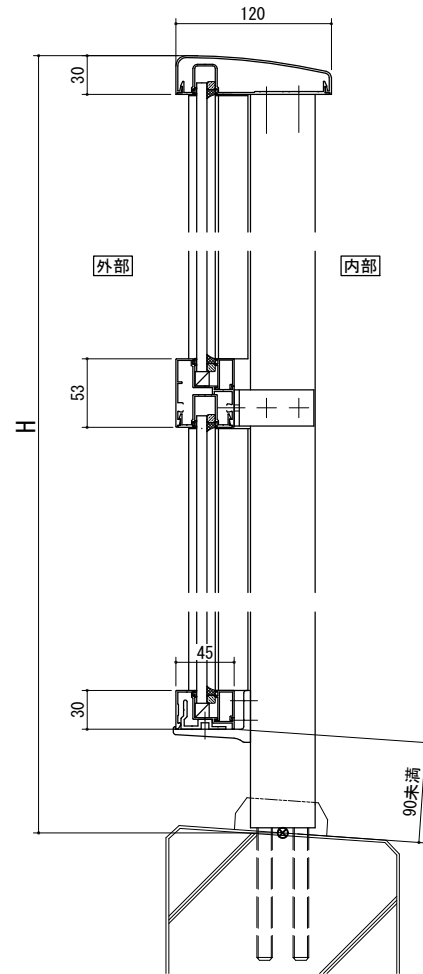
[上下ガラス堅枠Aタイプ] 端部
