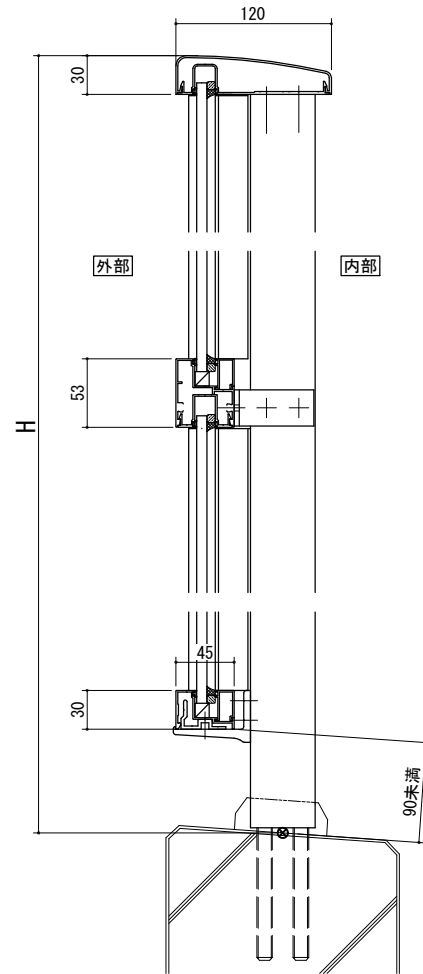
[上下ガラス堅枠Bタイプ] 端部
