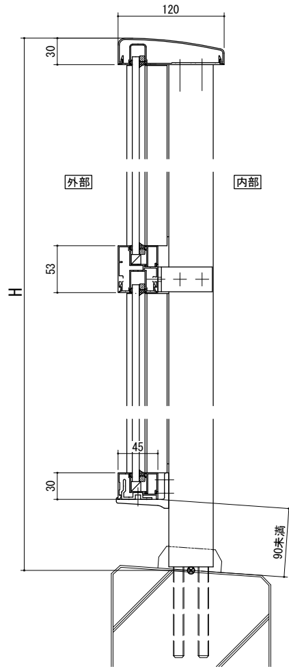
[上下ガラス堅枠Bタイプ] 中間
