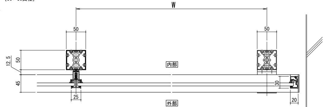
[50 x 50支柱]
