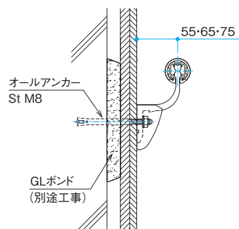
コンクリート下地 GL工法+PB2枚貼り
