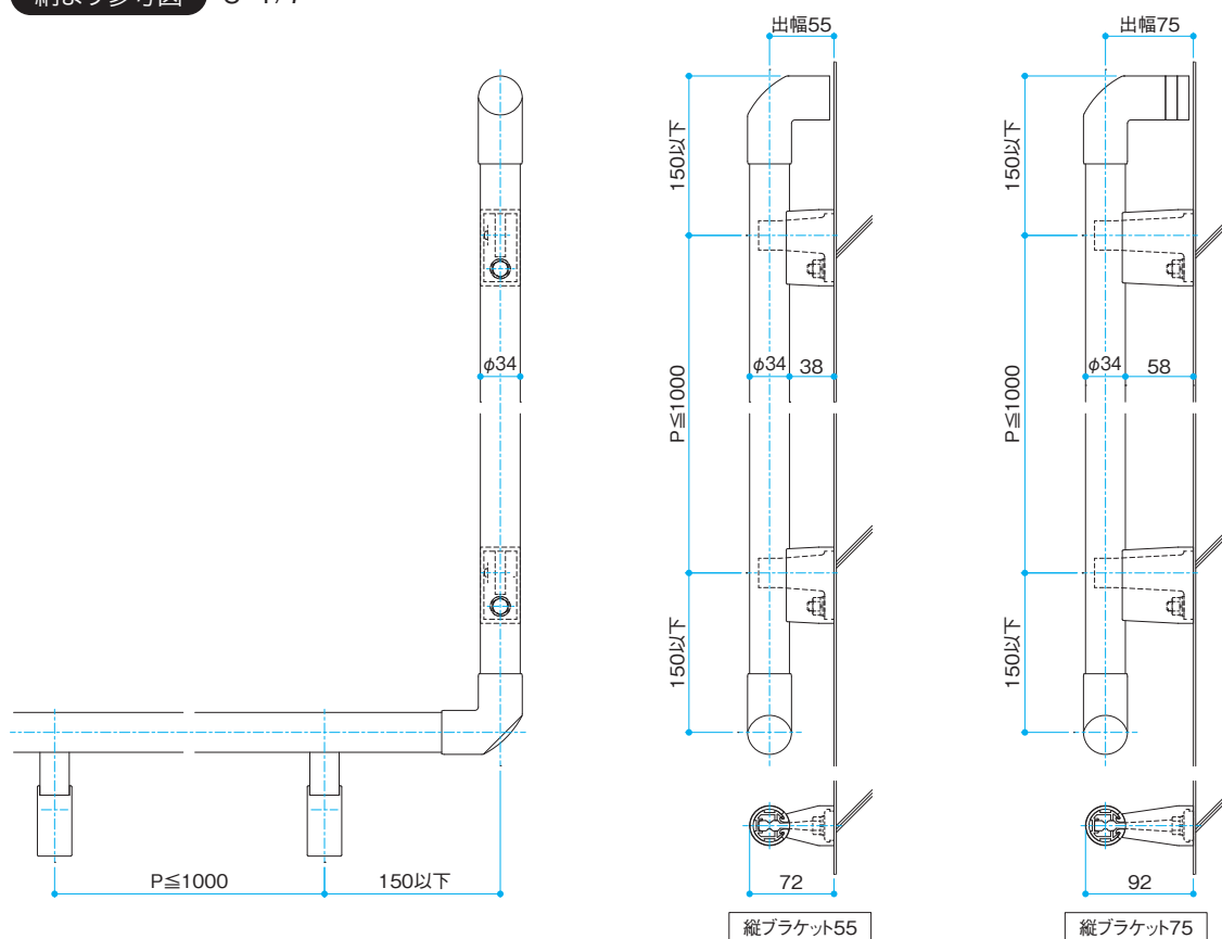
納まり参考図 S=1/7
