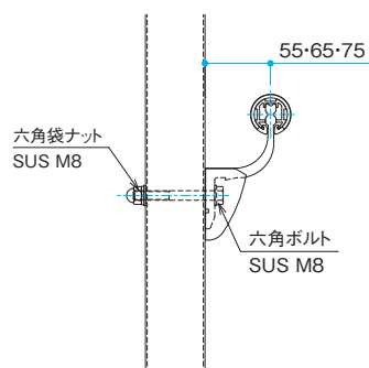
アルミ面取り合い (貫通ボルト)
