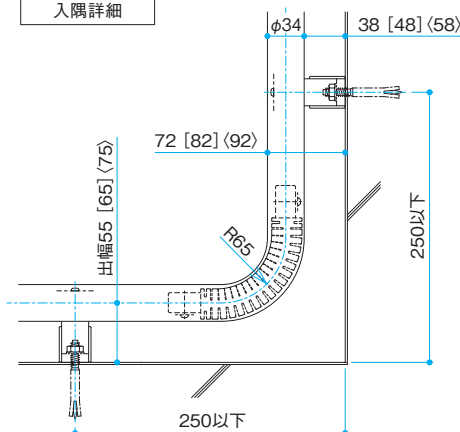
入隅詳細
