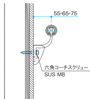
LGS (軽量鉄骨) 下地+木補強材
