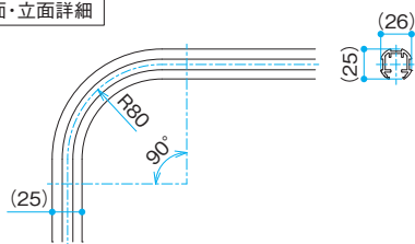
平面・立面詳細
