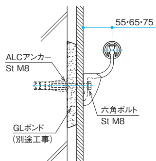
ALC下地+PB1枚貼り
