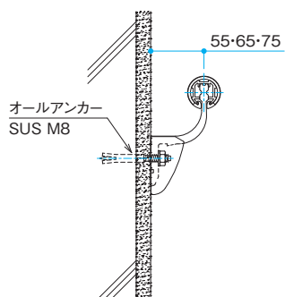
コンクリート下地
