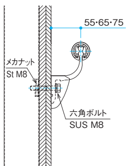
LGS (軽量鉄骨) 下地+PB2枚貼り
