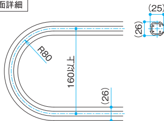
平面・立面詳細
