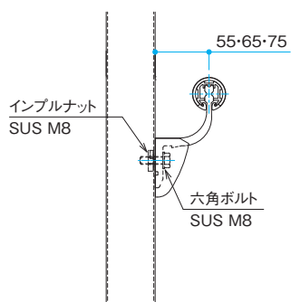
アルミ面取り合い (インプルナット)
