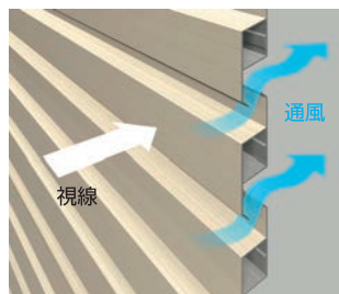
ガラリ部断面
