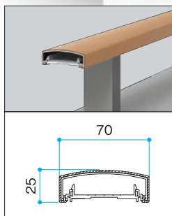
ハイブリッドファイン手すり70
