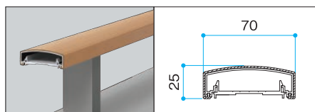
ハイブリッドファイン手すり70
