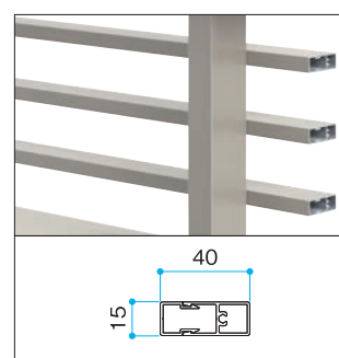
スリム横格子アウト
