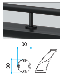
丸支柱φ30 丸手すりφ50用アーム
