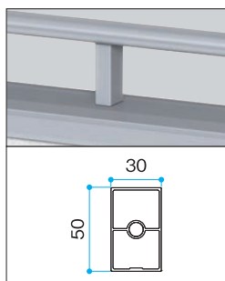
支柱30×50(エボリューション)
