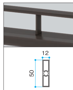
支柱12×50(エボリューション)
