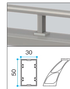
支柱30×50 楕円手すり80用アーム
