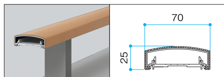
ハイブリッドファイン手すり70
