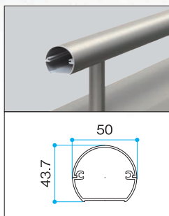
丸手すりφ50
