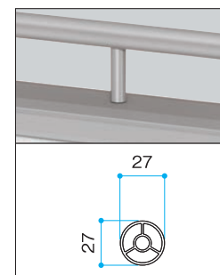
丸支柱φ27(エボリューション)
