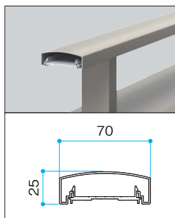
アルミファイン手すり70
